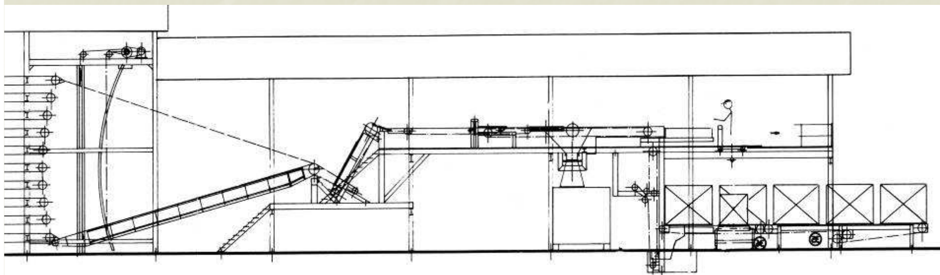
Vodorovné třídící boxy - vyprazdňování pomocí kyvného dopravníku
