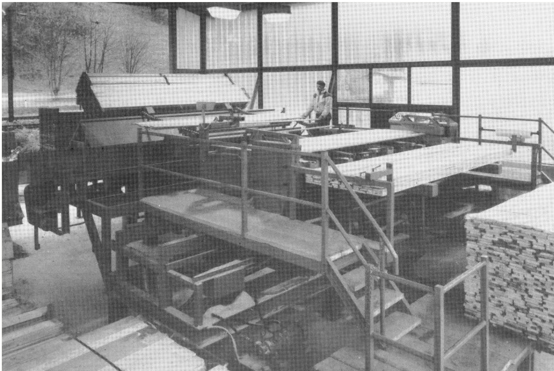
Rozebírací a ukládací zařízení
