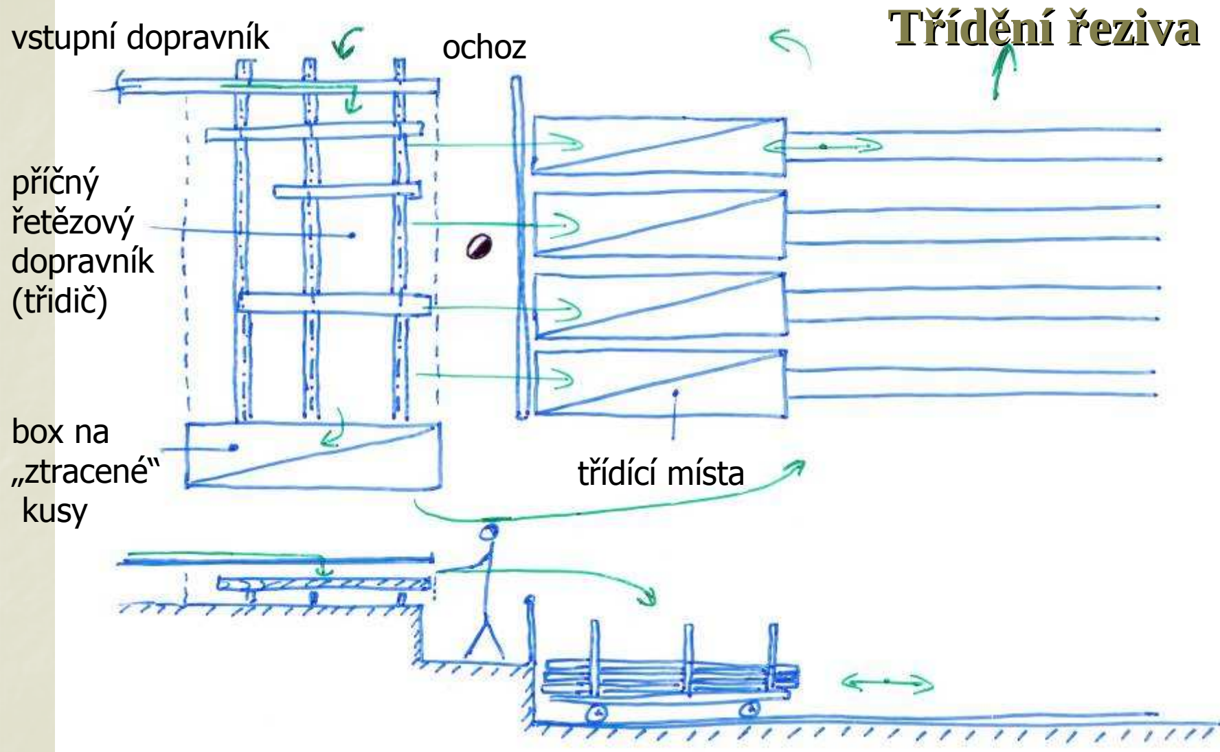
příčný řetězový třidič - na jednotlivé kusy řeziva
