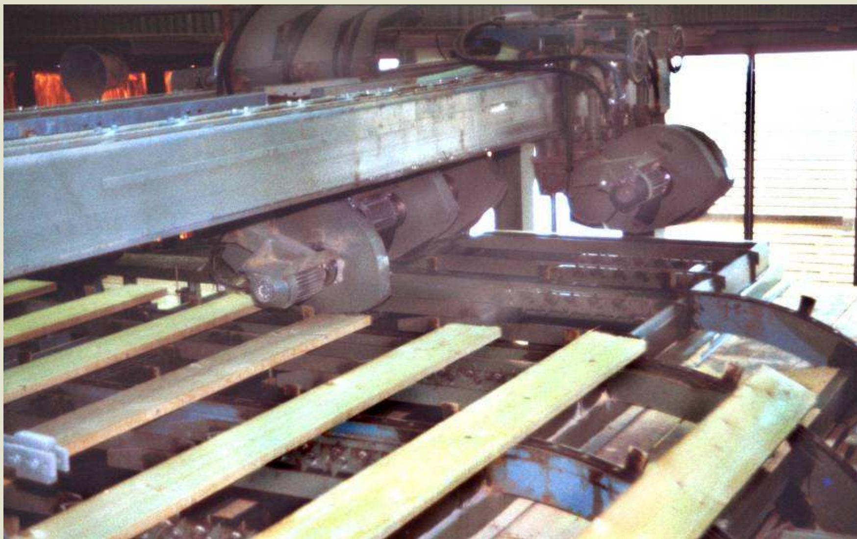
Krácení a kapování řeziva trimmerem před tříděním
